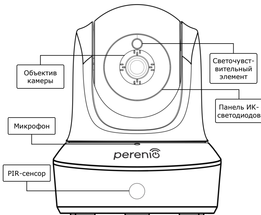
Рисунок 1 – Вид спереди
