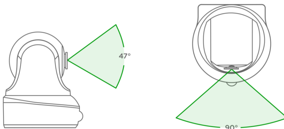
Рисунок 3 – Углы обзора
