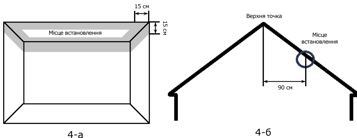
Малюнок 4 – Встановлення датчика диму на плоскій/скошеній стелі
