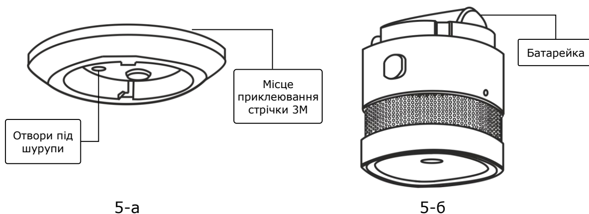
Малюнок 5 – Кріплення датчика диму на дюбелі або стрічку 3М
