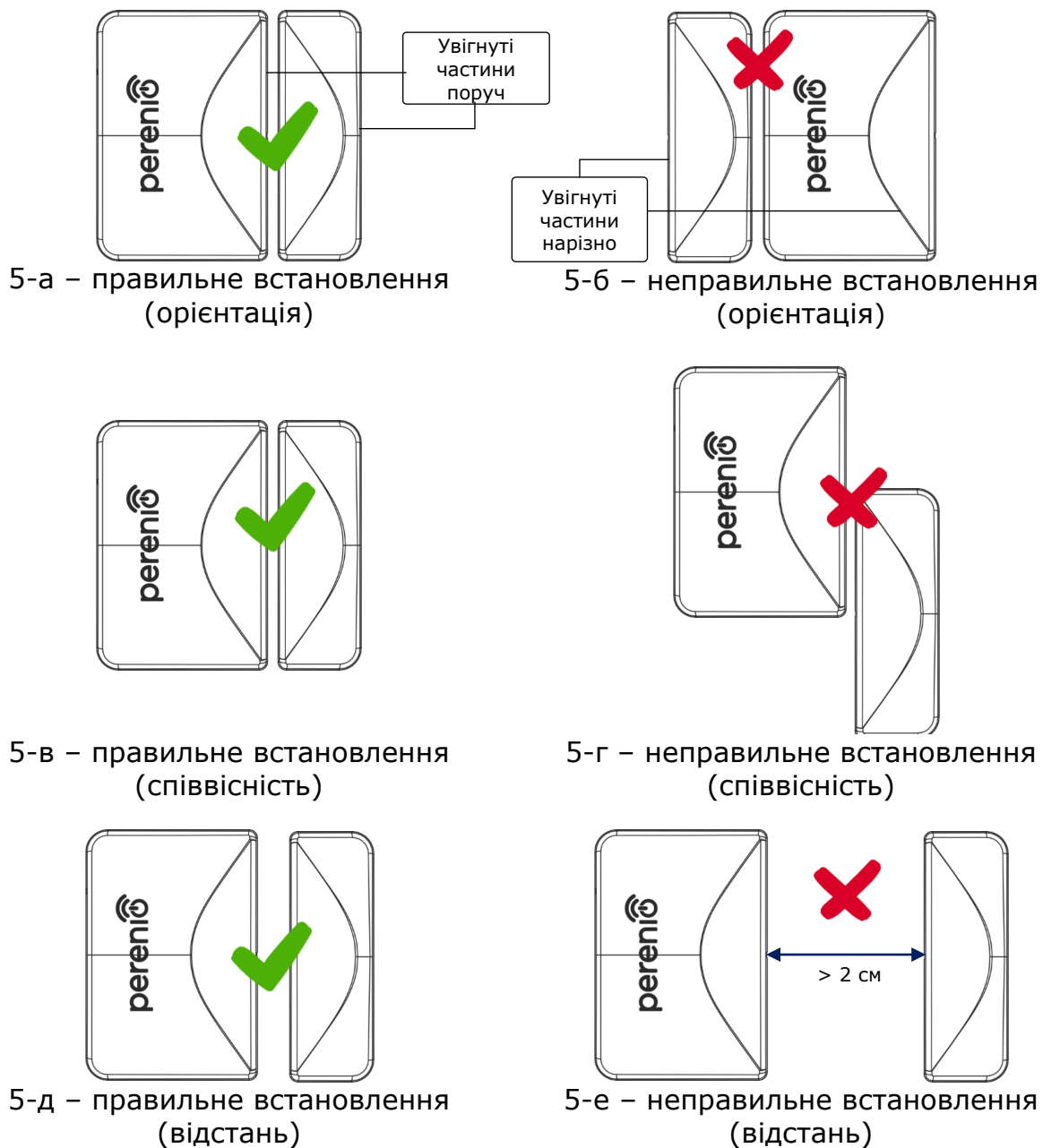
Малюнок 5 – Правила встановлення датчика та магніту
