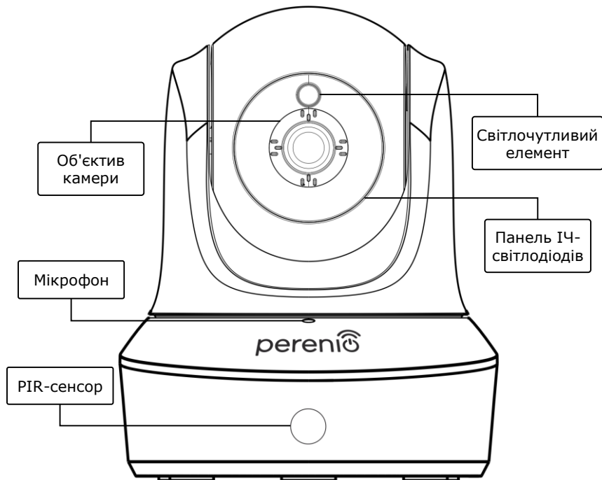
Малюнок 1 – Передня панель
