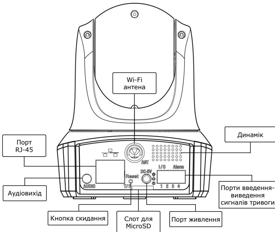
Малюнок 1 – Передня панель
